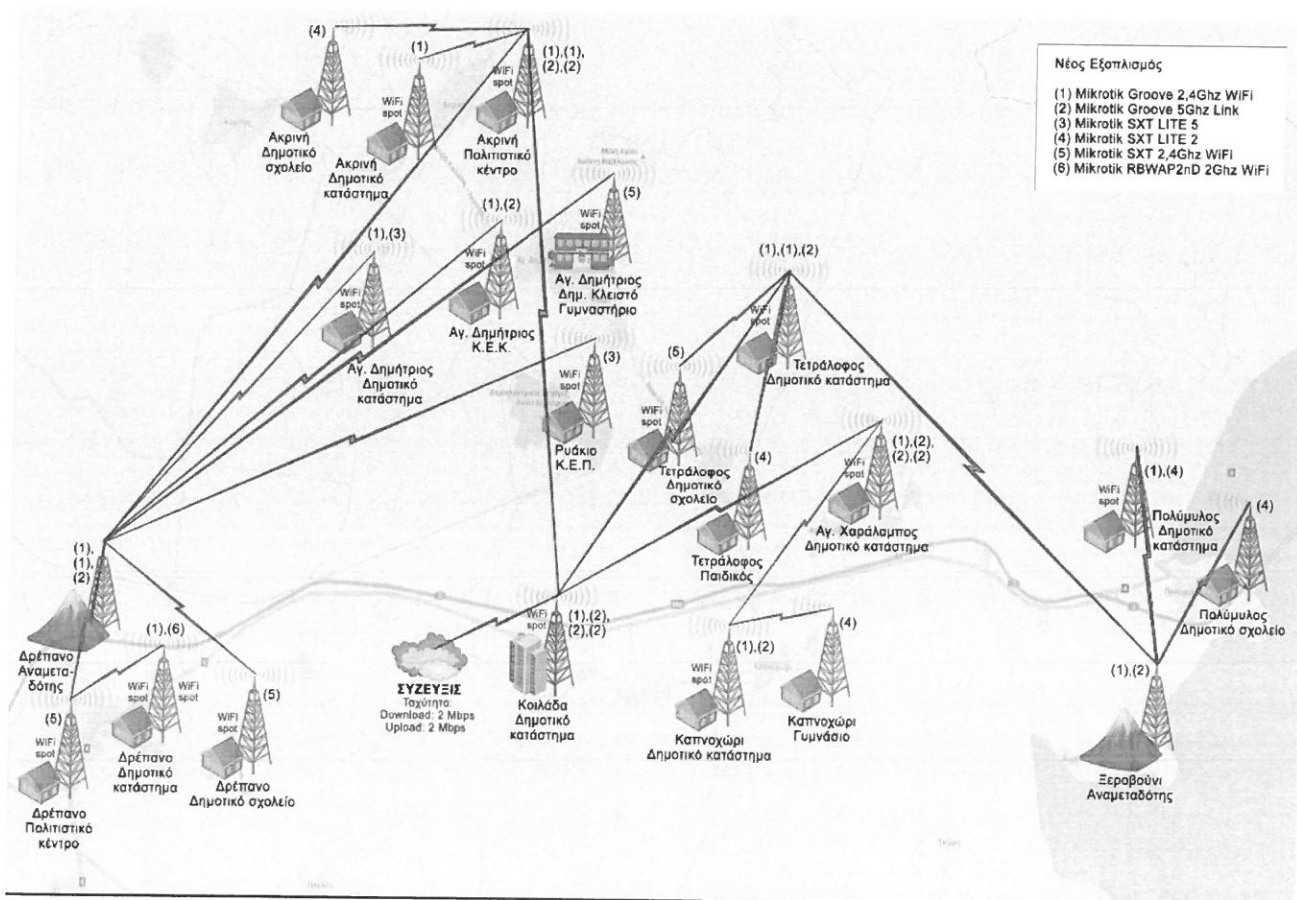
Σχήμα 1. Τοπολογία Ευρυζωνικού Δικτύου Δημοτικής Ενότητας Ελληνσπόντου
