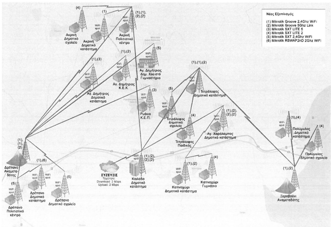
Σχήμα 1. Τοπολογία Ευρυζωνικού Δικτύου Δημοτικής Ενότητας Ελλησπόντου
